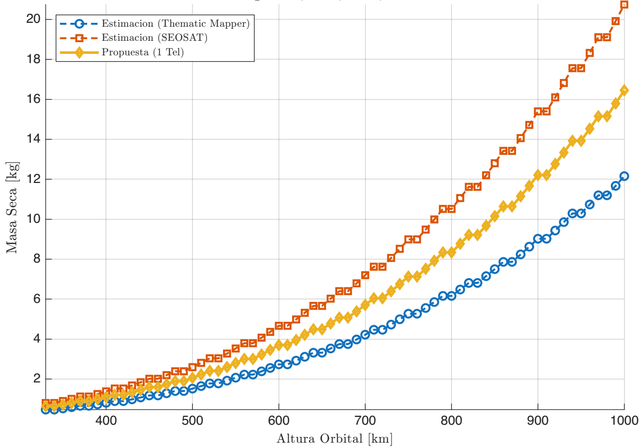
Comparativa de Masa Seca vs. Altura Config: 2 Sat, 1 Tel, Det 1, Refractivo
